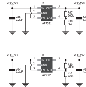
LDO
